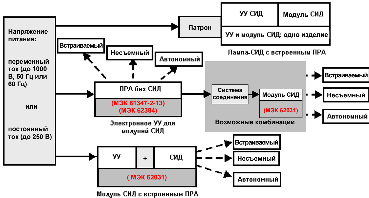
Рисунок В.1 – Обзор систем из модулей СИД и УУ
